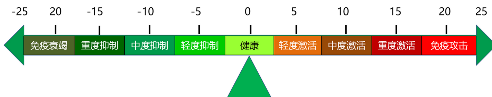
注: 0 分为免疫平衡状态,负分为免疫抑制,正分为免疫激活
